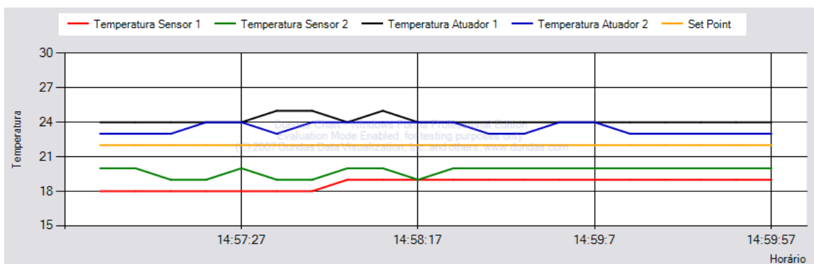
Figura 17- gráfico de temperaturas exibido em tempo real no software supervisorio.
