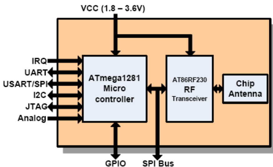
Figura 6- módulo ZigBit [8].
