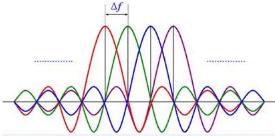
Figura 2.1: Subportadoras ortogonais em um sistema OFDM.
