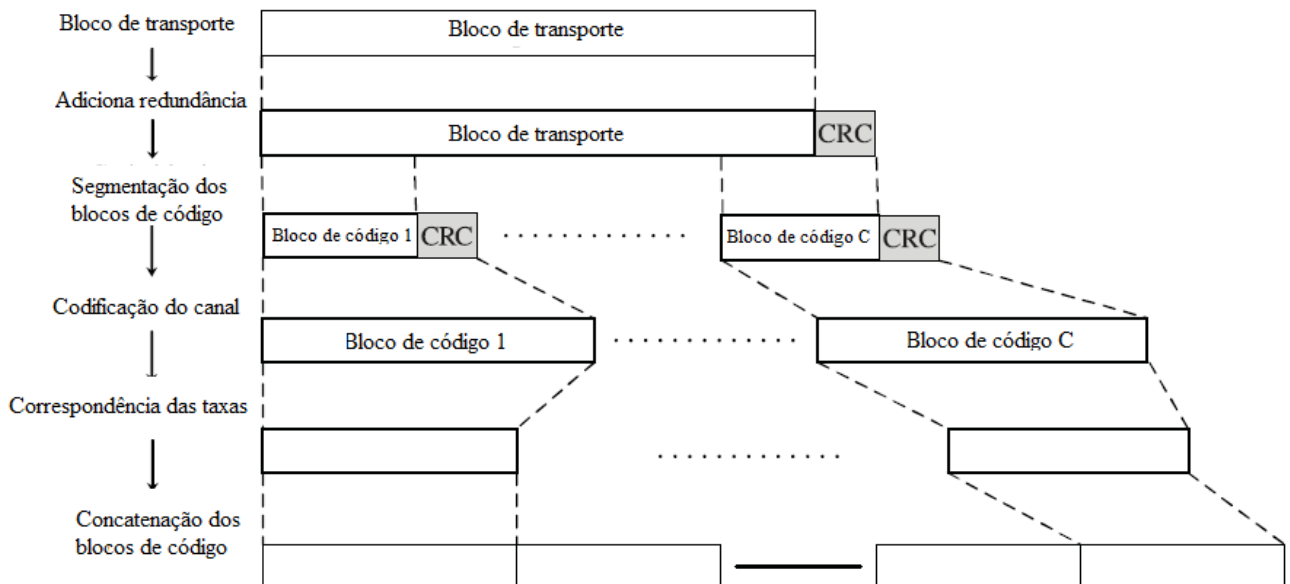
Figura 4.7: Processamento de codificação do canal [10].
