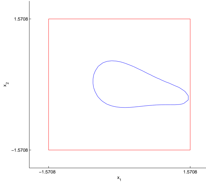
Figura 4.7: Estimativa do domínio de atração do Exemplo 2.2.2 com \lambda = 20 para o Teorema 5, curva em azul, e domínio C para a qual o sistema é localmente assintoticamente estável para o Resultado Principal (Proposto), em vermelho
