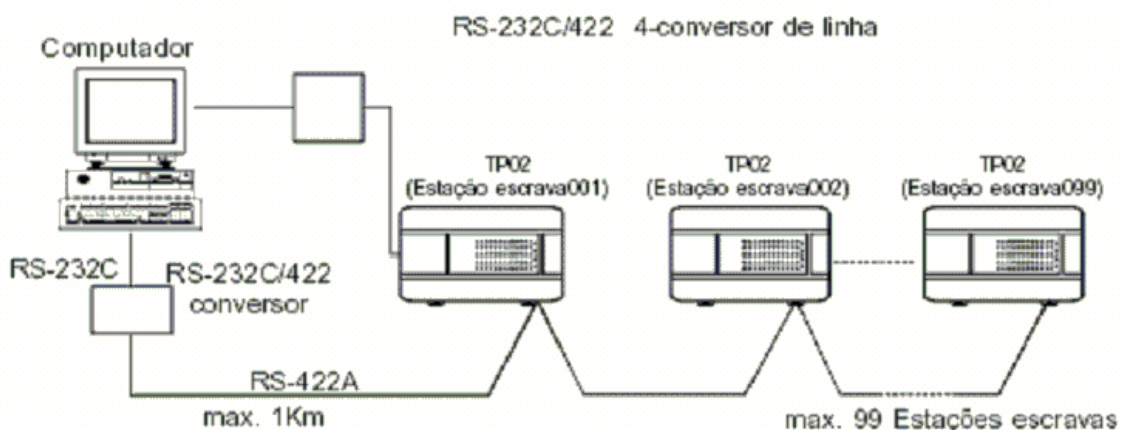
Figura 6.1 - Barramento Mestre-Escravo comandado pelo PC
