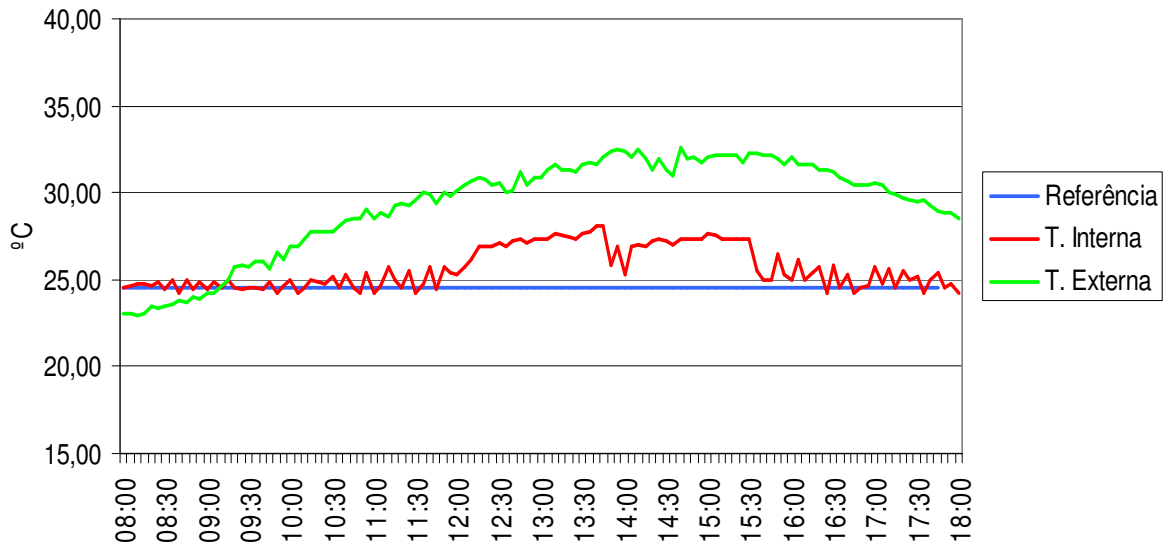
Figura 6.15 - Temperatura na Sala Diretoria – Controle fuzzy 14-09-2006
