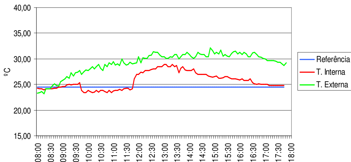
Figura 6.18 - Temperatura na Sala Reunião – Liga-Desliga 16-09-2006
