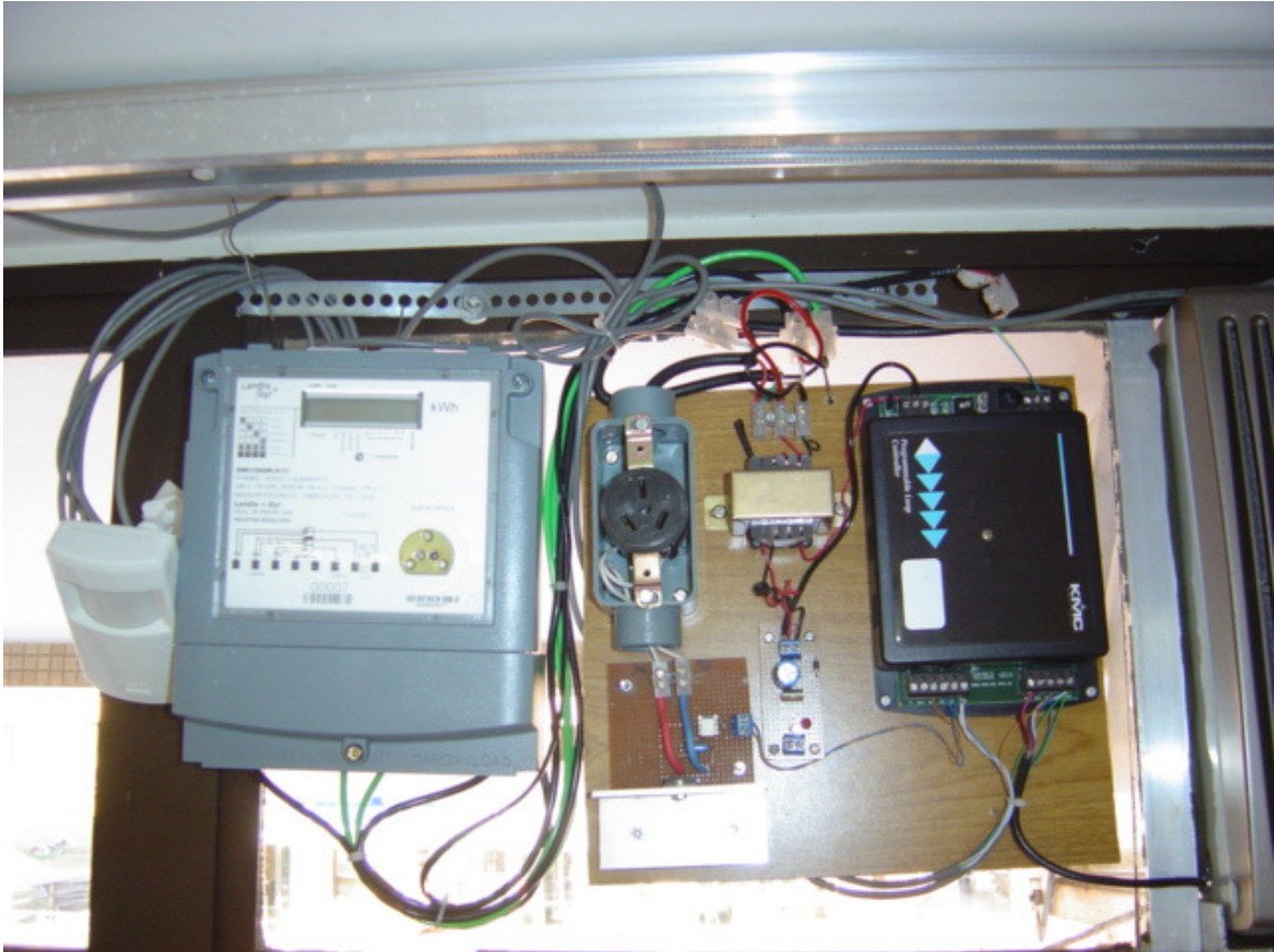
Figura 6.2 – Protótipo controlador predial distribuído
