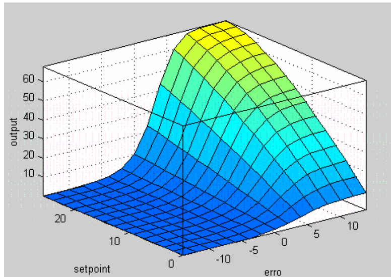
Figura 6.8 – Relação entre erro, referência e saída output.
