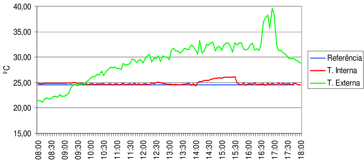
Figura 6.13 - Temperatura na Sala Desenvolvimento - Controle Fuzzy 14-09-2006
