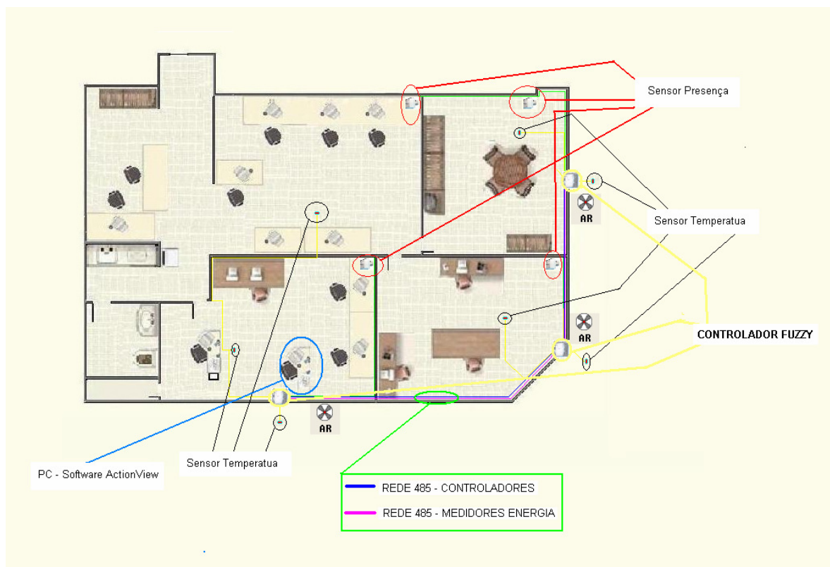
Figura 6.10 – Disposição dos sensores e equipamentos
