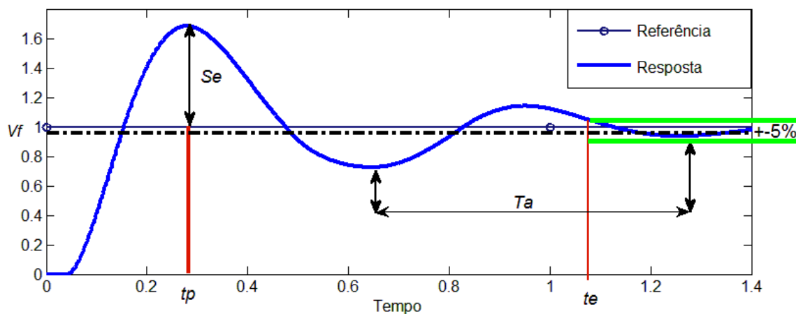
Figura 2.3: Parâmetros da resposta de sistema de controle genérico ao degrau unitário.
