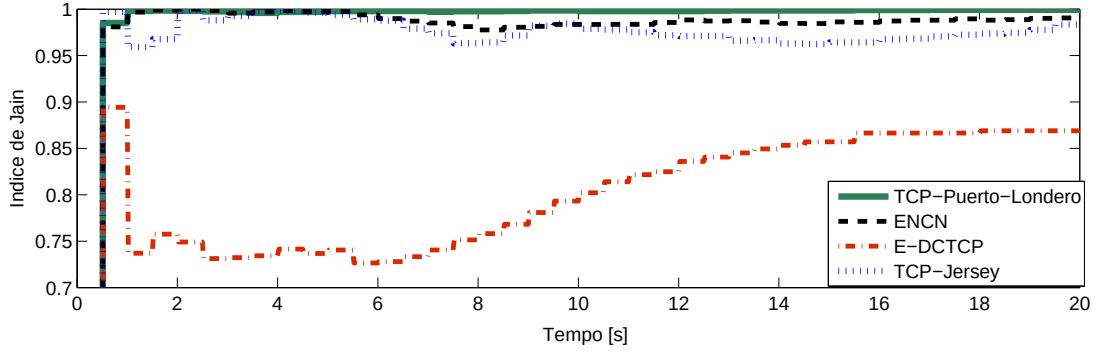
Figura 5.31: Índice de Jain para diferentes protocolos, implementados na topologia de rede de comunicação ilustrada na Figura 4.23.
