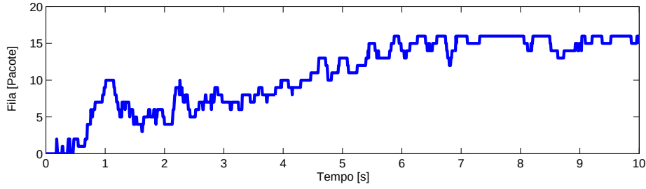
Figura 5.17: Fila no roteador 2 no sentido contrário ao fluxo TCP-Puerto-Londero.
