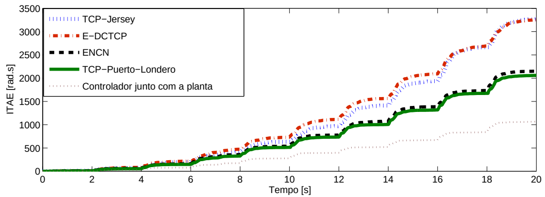
Figura 5.29: ITAE para diferentes protocolos, implementados na topologia de rede de comunicação ilustrada na Figura 4.23.
