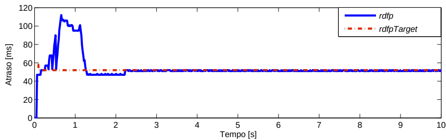
Figura 5.9: Atraso relativo no caminho de ida.
