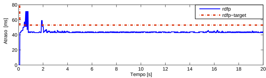
Figura 5.6: Atraso relativo no caminho de ida.
