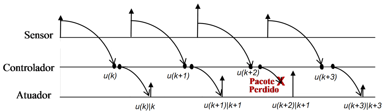
Figura 5.23: Possíveis casos para o controlador PI baseado em pacotes.
