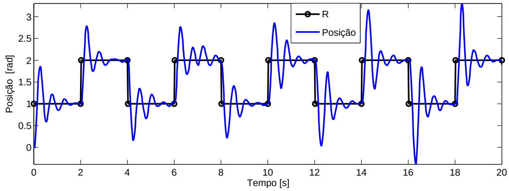
Figura 5.25: Posição do motor com perturbação de 3 V aplicado aos 7 s, compartilhando a mesma topologia de rede com fluxos TCP-Jersey
