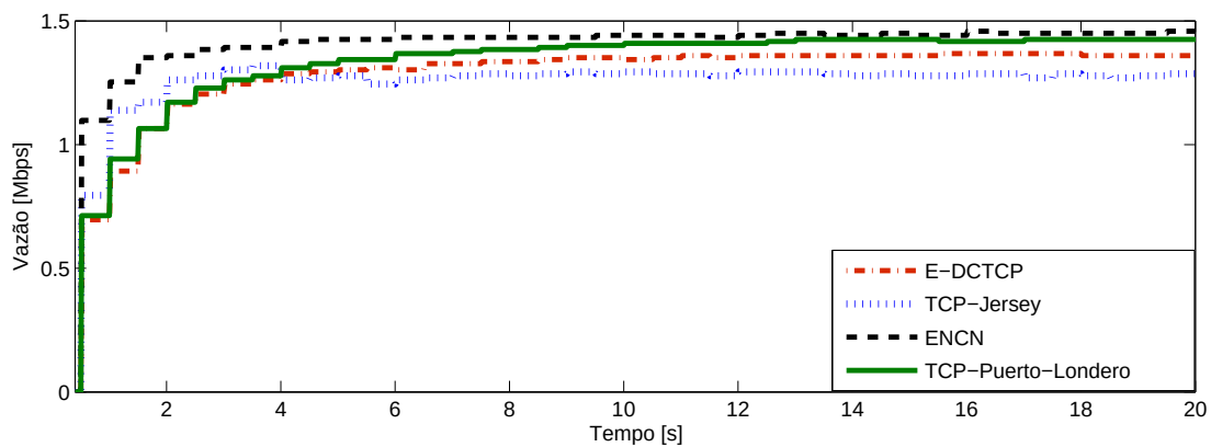
Figura 5.30: Vazão para diferentes protocolos, implementados na topologia de rede de comunicação ilustrada na Figura 4.23.
