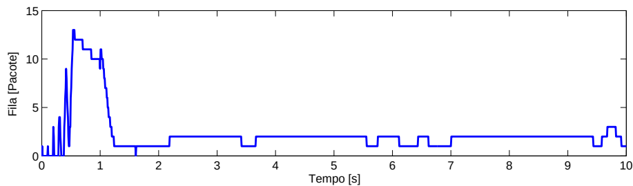
Figura 5.16: Fila no roteador 1 no sentido do fluxo TCP-Puerto-Londero na presença de congestionamento no caminho de retorno.
