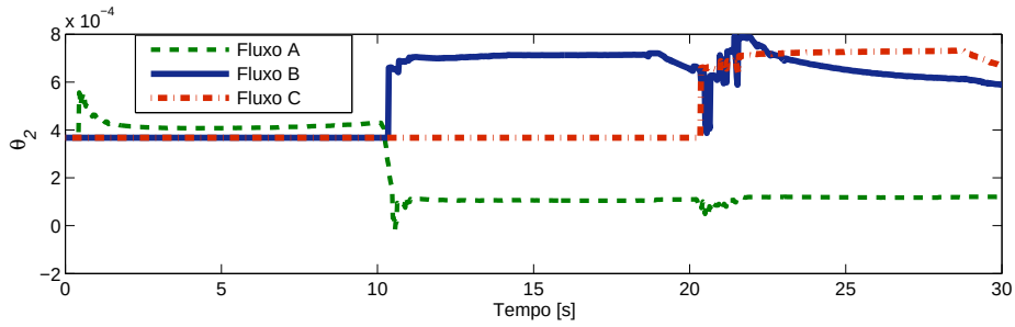
Figura 5.19: Readaptação do parâmetro \theta_2 em cada fluxo TCP-Puerto-Londero.
