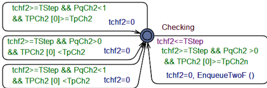
Figura I.7: Modelo do canal 2 de ida.
