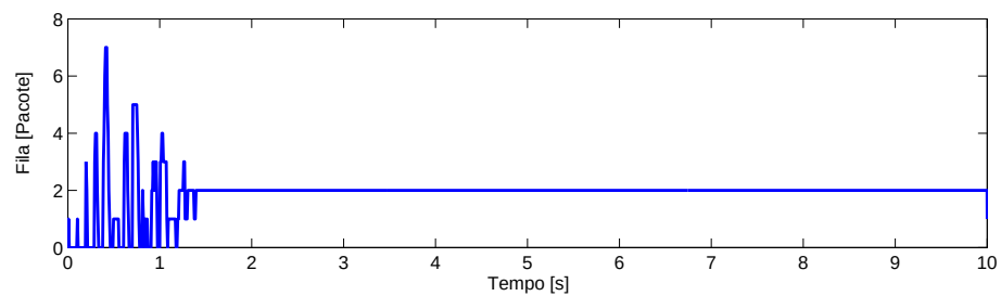
Figura 5.5: Fila no caminho de ida gerada pelo controlador nominal.
