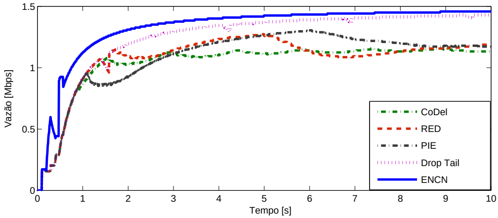
Figura 4.5: Vazão de ENCN comparada com outras técnicas AQM, implementadas na topologia de rede de comunicação dada na Figura 3.3.
