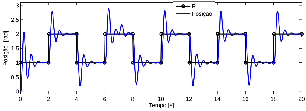
Figura 5.27: Posição do motor com perturbação de 3 V aplicado aos 7 s, compartilhando a mesma topologia de rede com fluxos ENCN.
