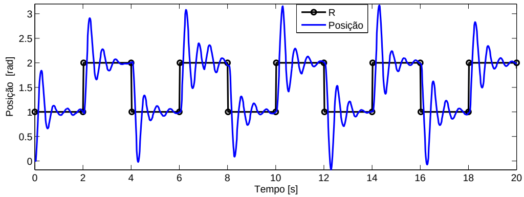
Figura 5.26: Posição do motor com perturbação de 3 V aplicado aos 7 s, compartilhando a mesma topologia de rede com fluxos E-DCTCP.
