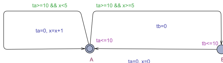
Figura 3.1: Simples autômato de dois estados em UPPAAL.
