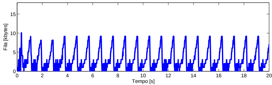
Figura 5.32: Fila para TCP-Jersey.
