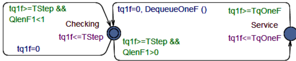
Figura I.5: Modelo da fila de dados no caminho de ida, no roteador 1.
