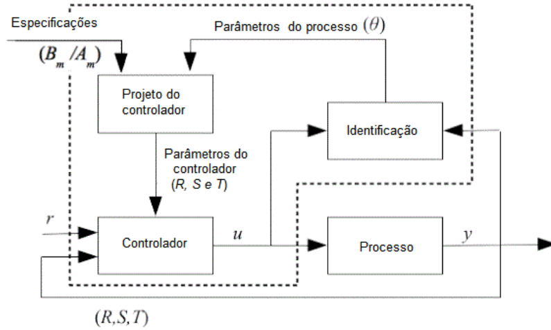
Figura 5.8: Diagrama em blocos do controlador adaptativo.
