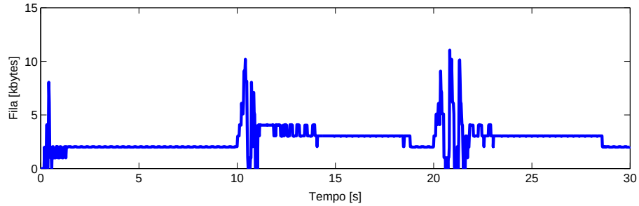
Figura 5.20: Fila no roteador 1 .
