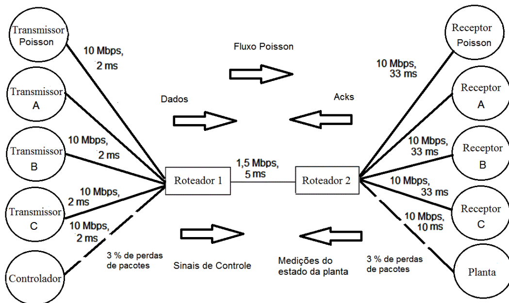
Figura 5.36: Topologia de rede de comunicação tipo Dumbbell com um tráfego de fundo compartilhada por três fluxos TCP e um fluxo UDP de uma NCS.
