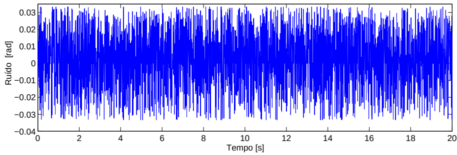
Figura 5.22: Ruído de medição colocado na saída da planta.
