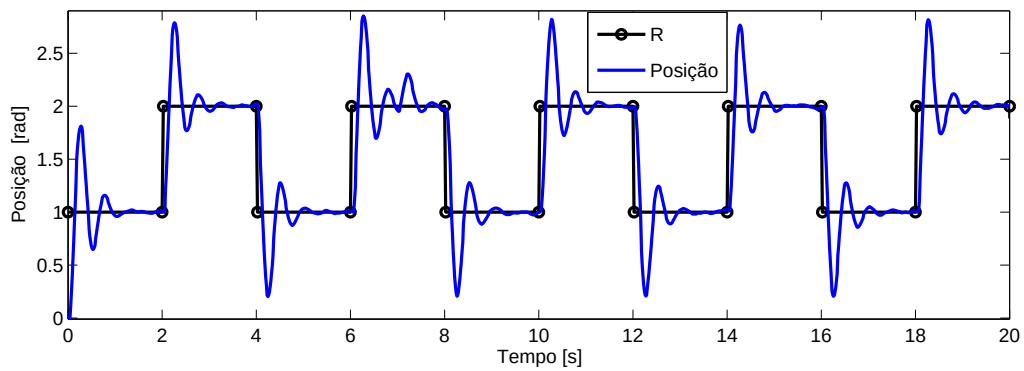
Figura 5.28: Posição do motor com perturbação de 3 V aplicado aos 7 s, compartilhando a mesma topologia de rede com fluxos TCP-Puerto-Londero.
