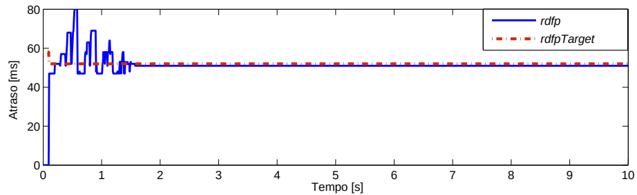
Figura 5.3: Atraso relativo no caminho de ida fornecido pelo controlador nominal.
