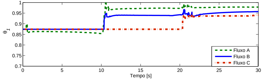
Figura 5.18: Readaptação do parâmetro \theta_1 em cada fluxo TCP-Puerto-Londero.
