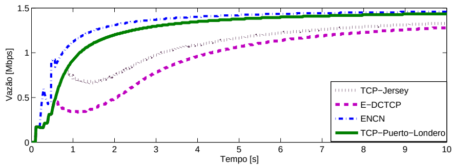
Figura 5.12: Fila no caminho de ida.
