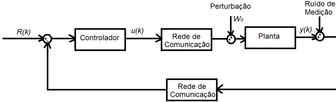
Figura 5.21: Malha de controle.
