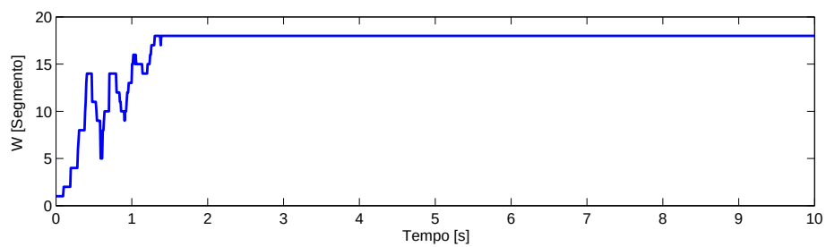
Figura 5.4: Janela de transmissão W obtida mediante o uso do controlador nominal.
