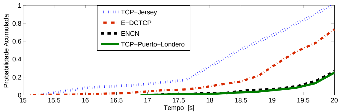
Figura 5.37: Probabilidade acumulada do ITAE ser maior que 3500,00 rad.s em até 20 s.
