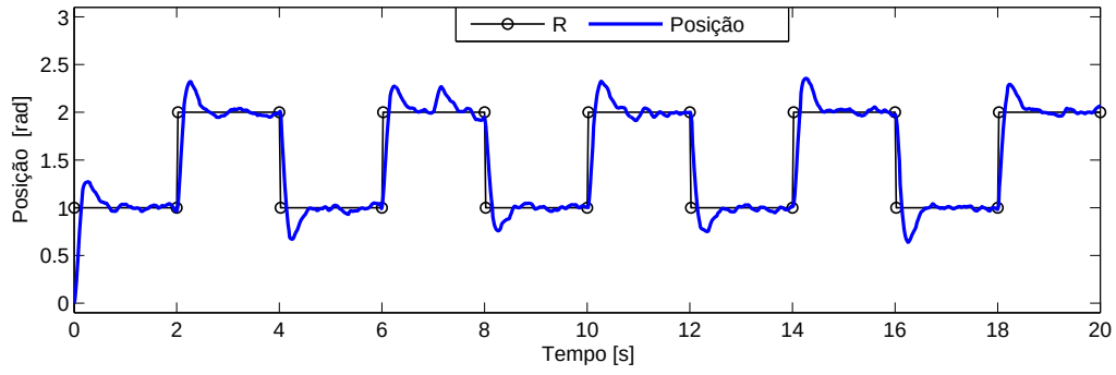
Figura 5.24: Posição do motor para o caso no qual o controlador está junto com a planta com perturbação de 3 V aplicado aos 7 s.
