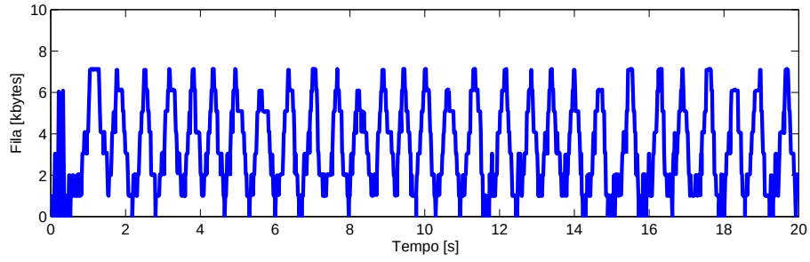
Figura 5.33: Fila para E-DCTCP.
