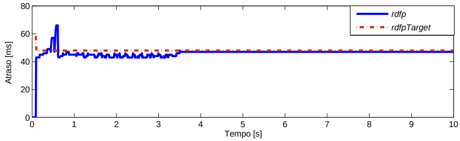
Figura 5.13: Atraso relativo no caminho de ida.
