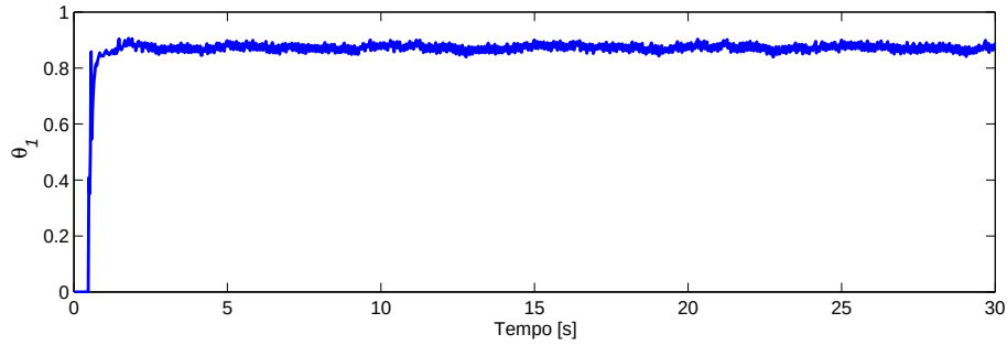
Figura 5.1: Parâmetro da função de transferência da topologia de rede de comunicação da Figura 3.3.
